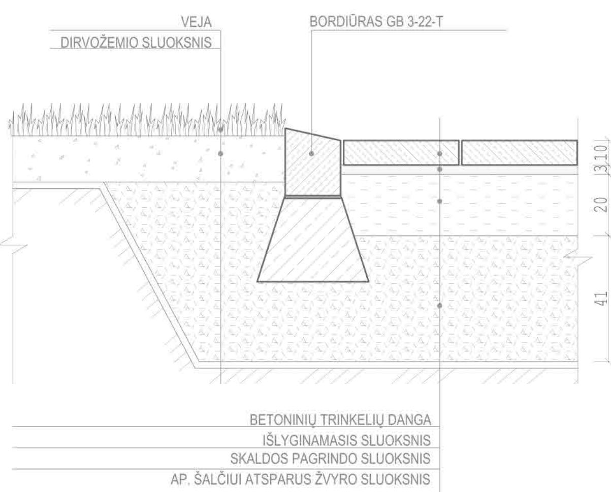
TRINKELIŲ DANGOS VAŽIUOJAMOJOJE DALYJE M 1:20
