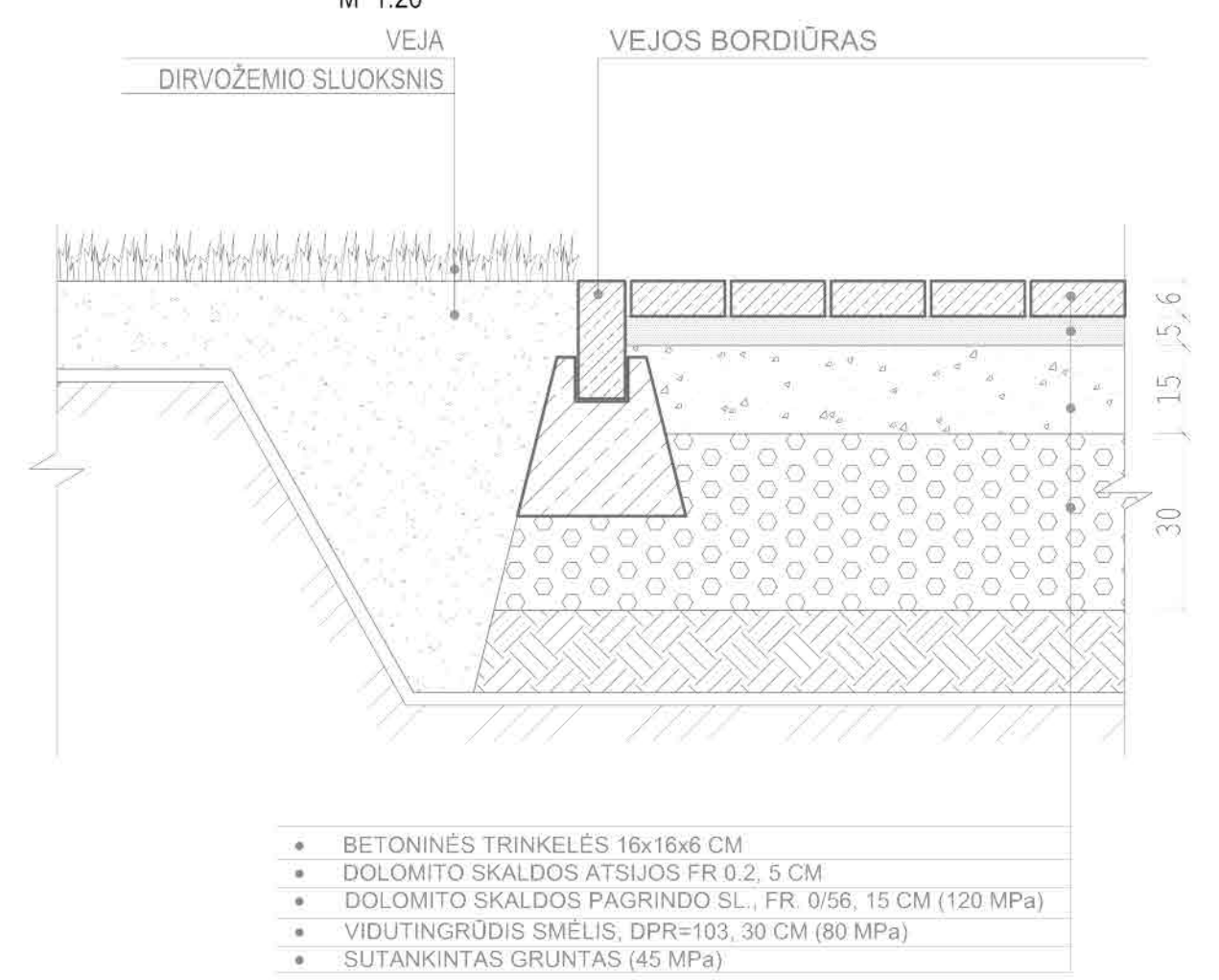
TRINKELIŲ DANGOS DETALĖ PĖSČIŲŲ ZONOJE M 1:20
