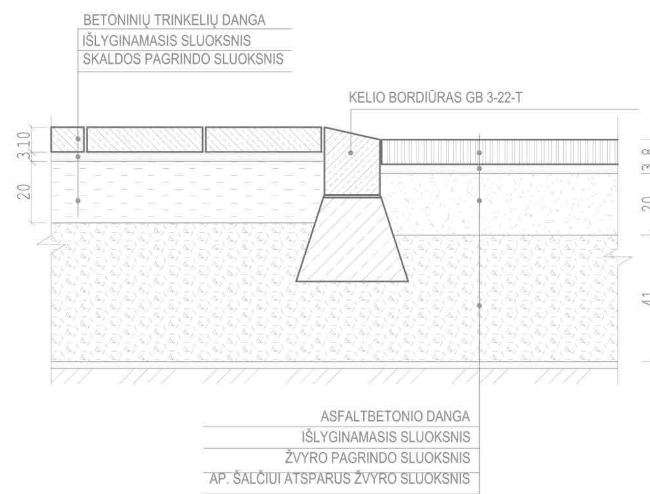
TRINKELIŲ IR ASFALTO DANGŲ DETALĖ M 1:20
