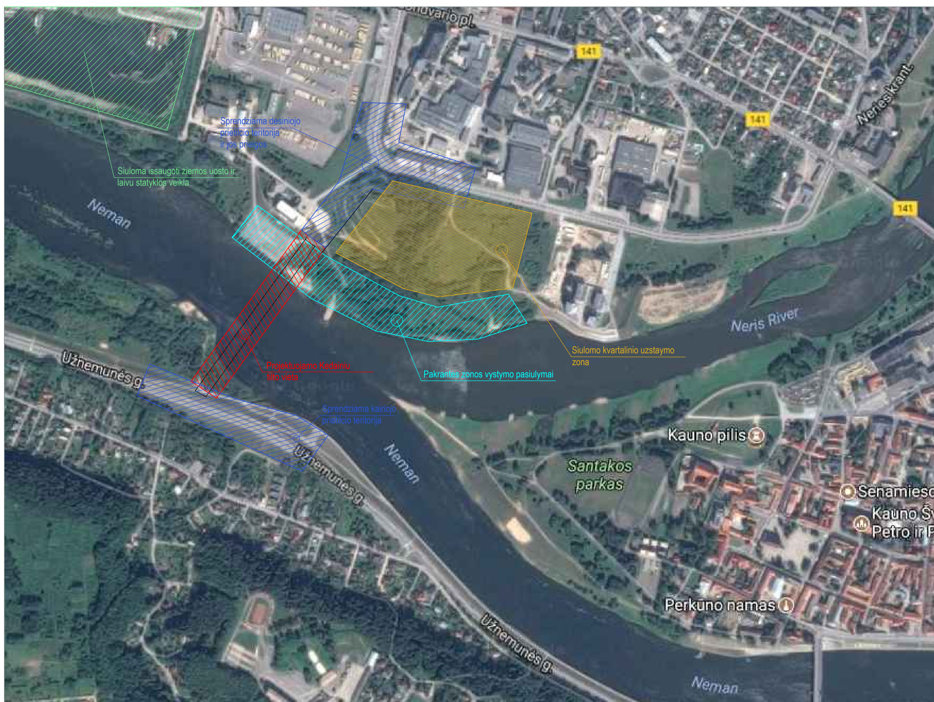
Tilto ir jo prieigų situacijos schema m 1 : 10 000
