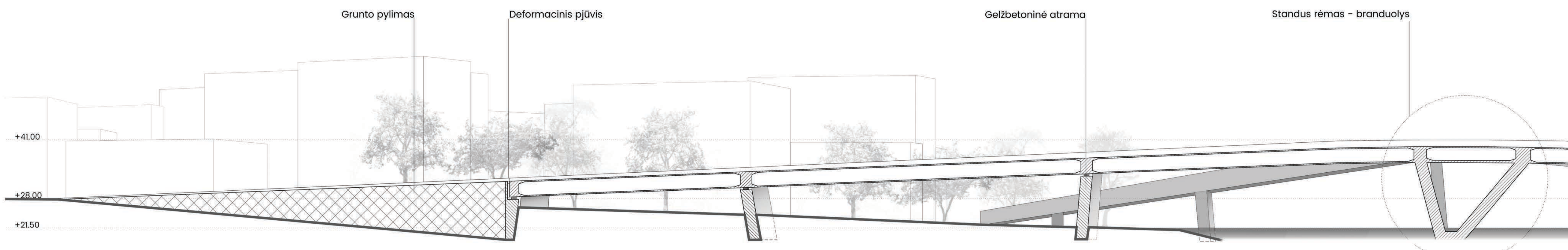
IŠILGINIS PJŪVIS M 1:500
