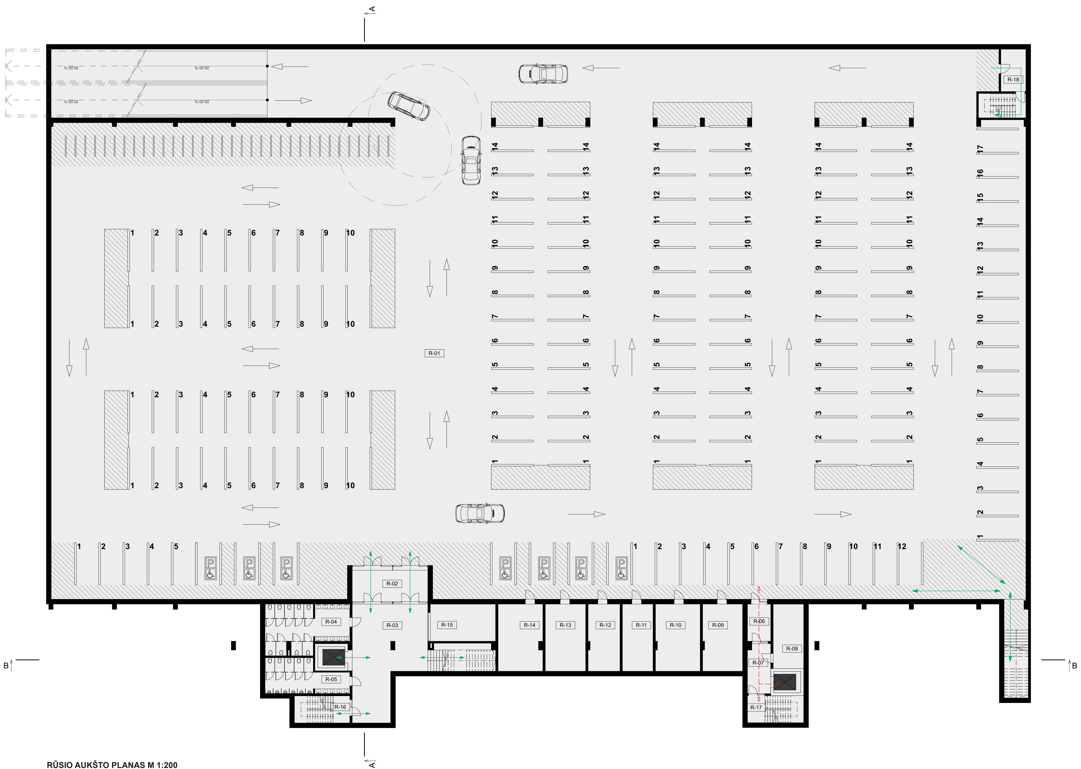
RŪSIO AUKŠTO PLANAS M 1:200
