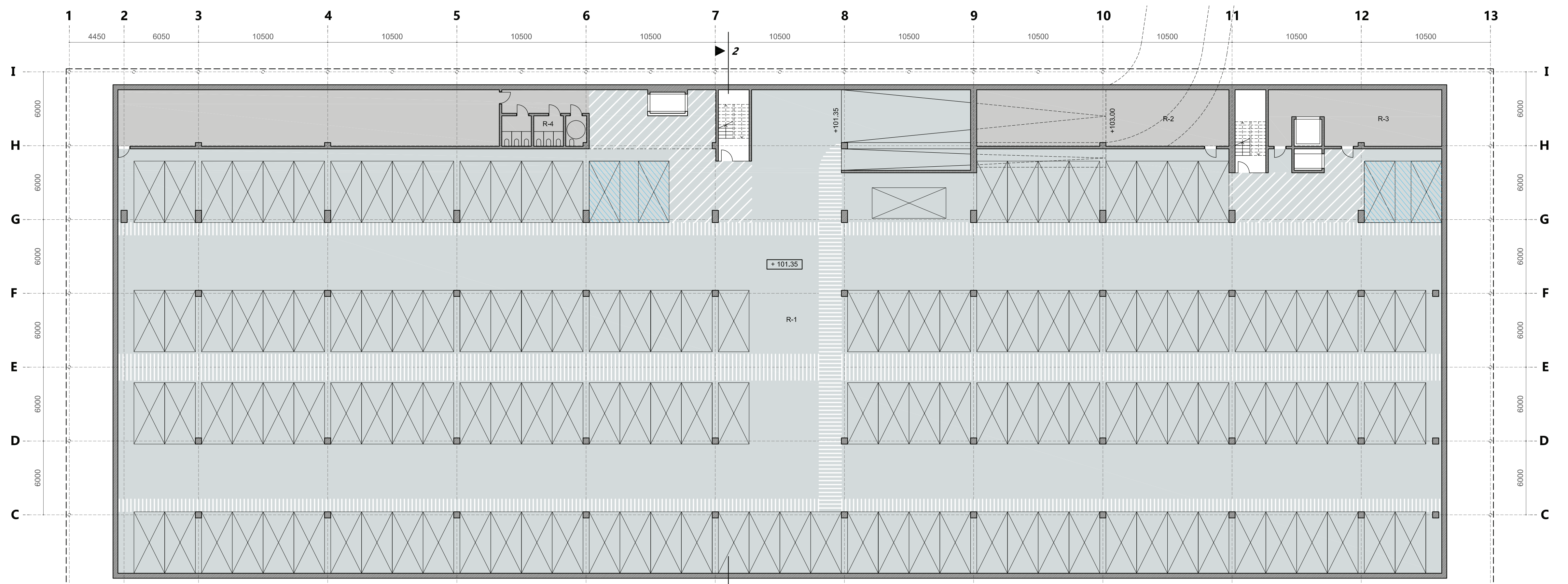
Rūšio aukšto planas M1:200
