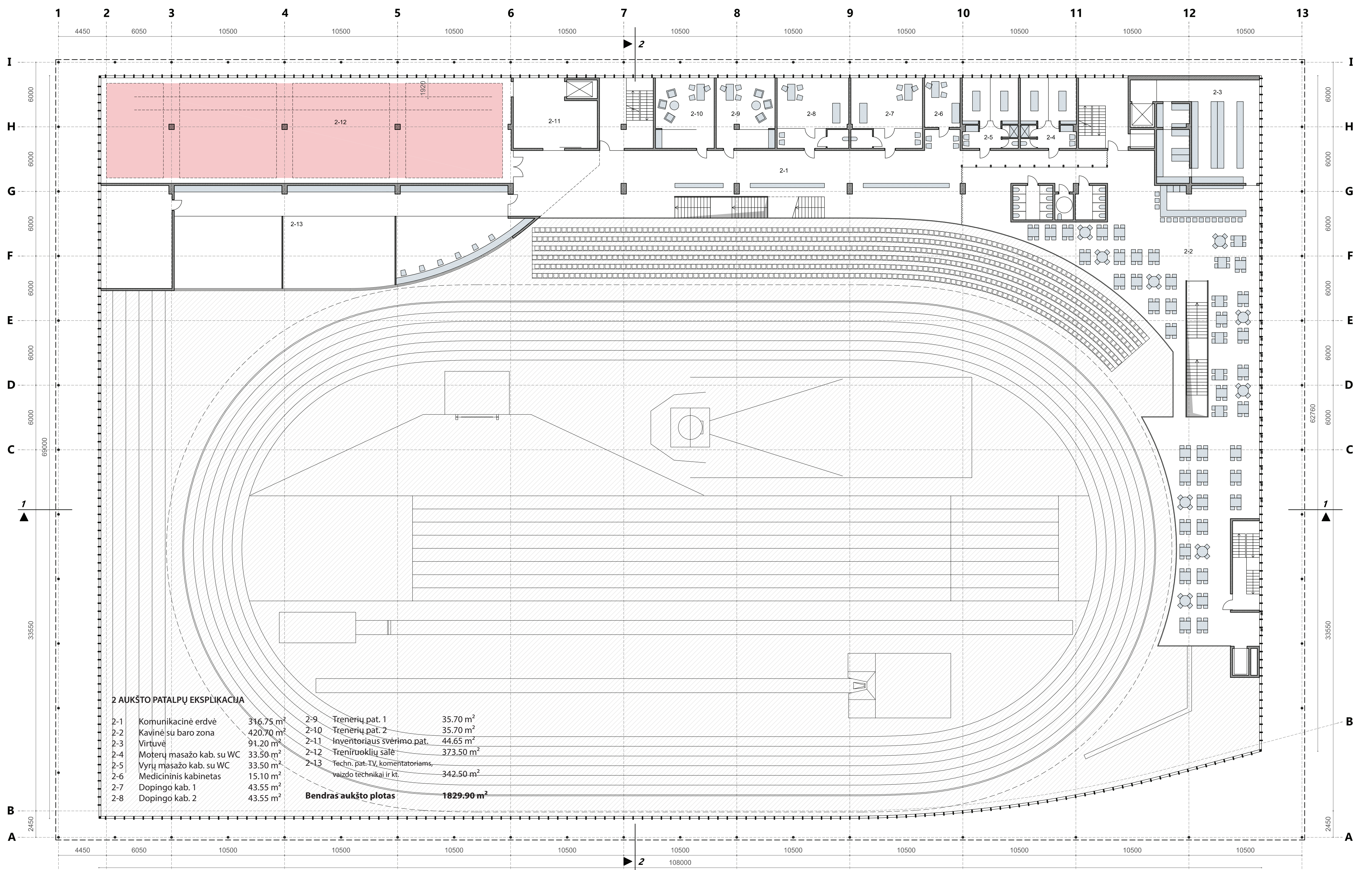
2 aukšto planas M1:200
