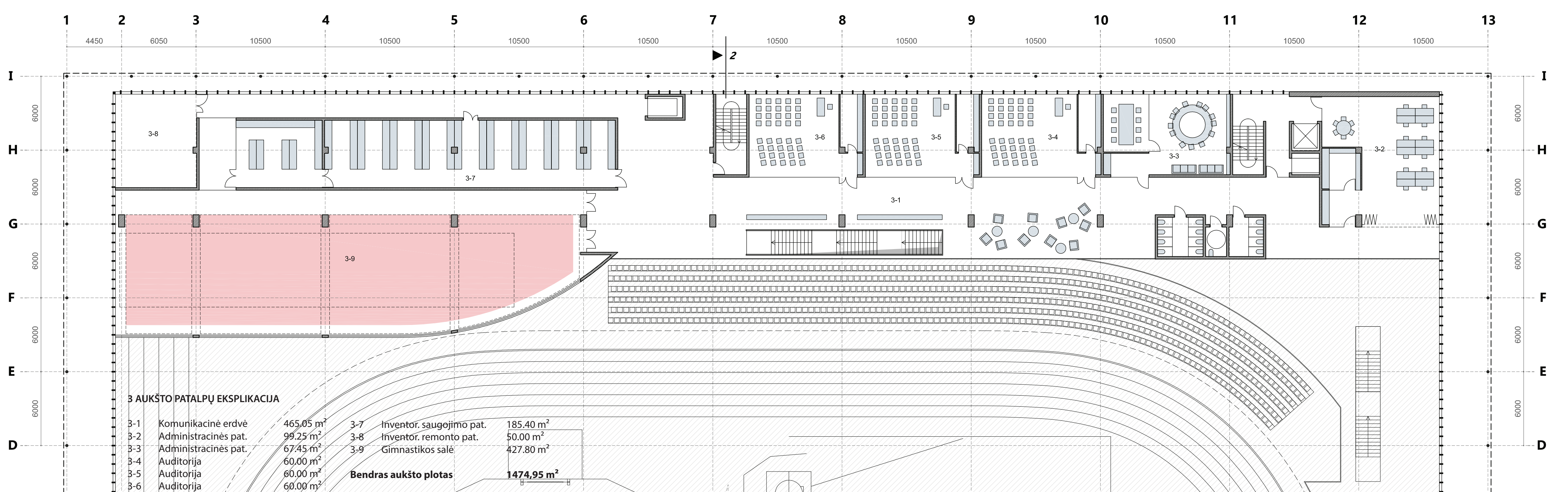
3 aukšto planas M1:200
